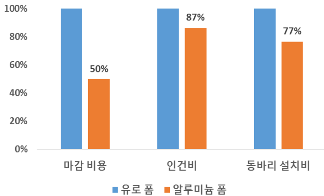
그림 3. 유로 폼 대비, 알루미늄 폼의 비용 비율
