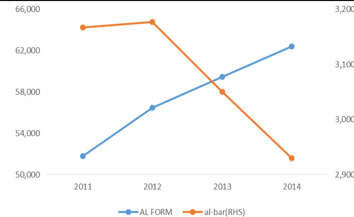
그림 31. 알루미늄 bar, 알루미늄 품 가격
