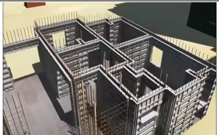
그림 2. Aluminum Form을 이용한 거푸집 모형
