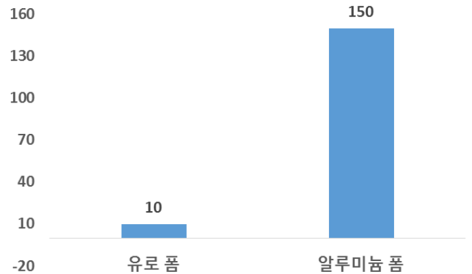
그림 4. 거푸집 별 최소 사용 가능 횟수 (단위: 회)
